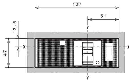
A=71 4 POLES
